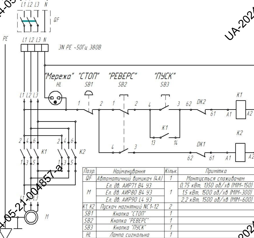
Рисунок 2.1 Схема електрична принципова МІМ-150, МІМ-300, МІМ-600
